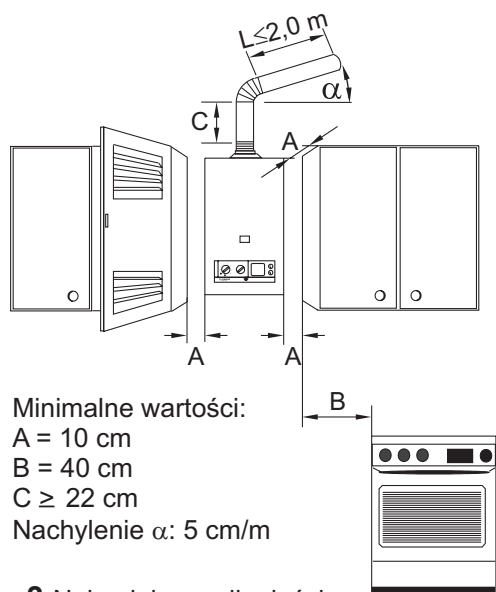
Rys. 3 Najmniejsze odległości przy zabudowie grzejnika
